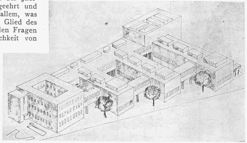
1. Rang, Entwurf Nr. 20. Fliegerbild aus Osten.
