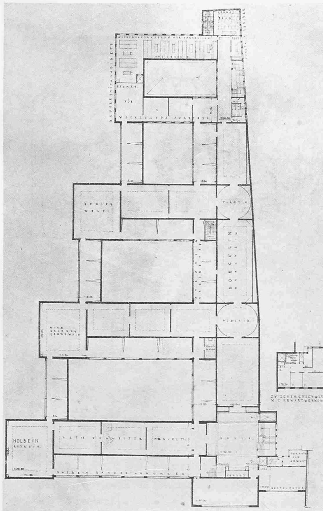
Entwurf Nr. 20. — Erstes Obergeschoss, 1:800.
