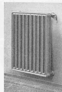
Abb. 1 und 2. „Columbus“-Radiatoren der v. Roll'schen Eisenwerke Klus.
