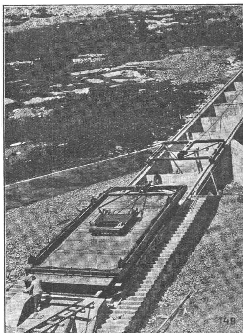
Schütze zum Stollenabschluss Wägital, max. Wasserdruck ca. 2300 t.
