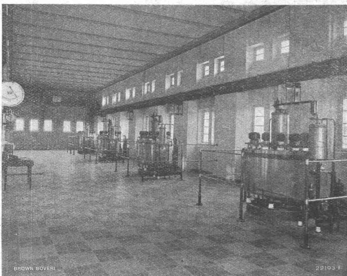
Gleichrichter-Unterstation Tegel der Deutschen Reichsbahn bestehend aus vier Gleichrichtergruppen zu je 400 kW bei 835 V Gleichstrom.
