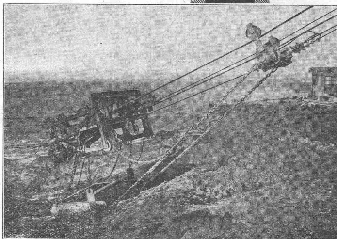
Kabelbagger-Laufkatze mit Kettenzaum und Schürfkübel von 4 m³.
