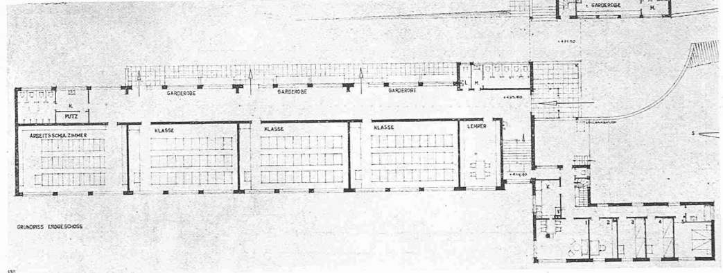
Abb. 4. Grundriss 1:500.
