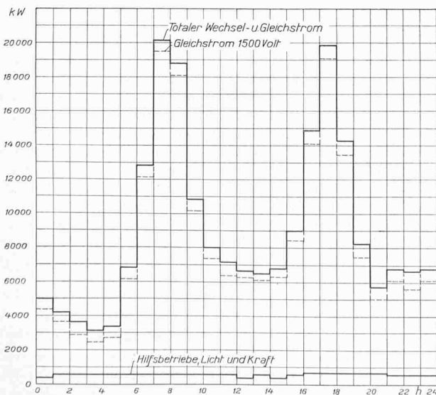
Abb. 1. 24-stündiges Belastungsdiagramm der Ill. C. R.
