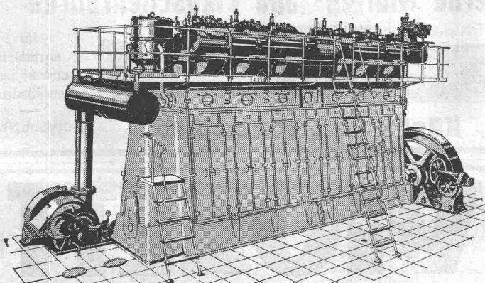
1700 PSe S. L. M.-Dieselmotor mit Büchi-Abgasturbinenaufladung
