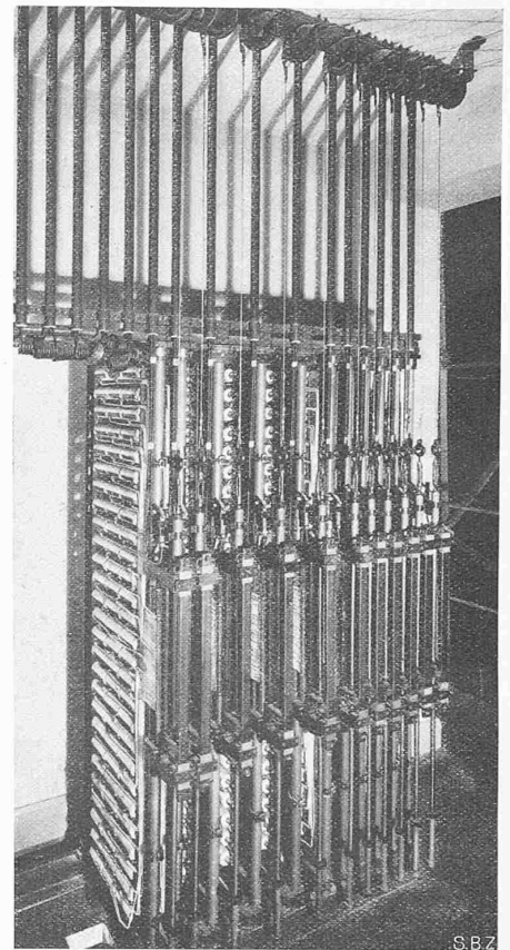
Abb. 27. Regulierwiderstände zum Stellwerk.
