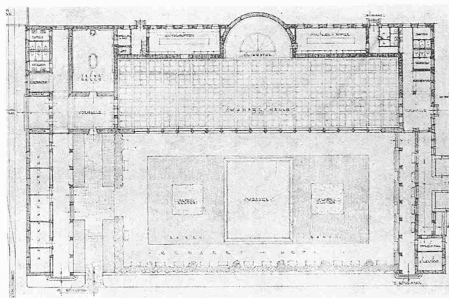
Oben: Grundriss 1:800. Nebenan: Lageplan 1:4000.
