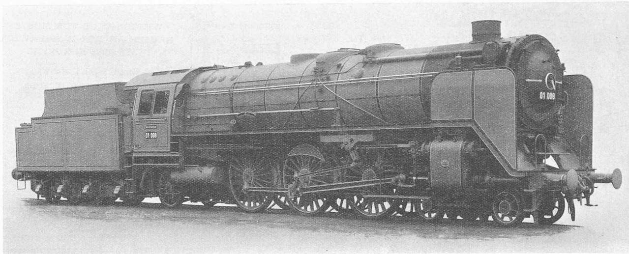
Einheits-Schnellzuglokomotive, Heissdampf-Zweizylinder-Zwillingsmaschine, Typ 2C1, der Deutschen Reichsbahn.
