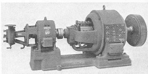
Abb. 7. Kühlgruppe für das Transformatoren-Oel.
