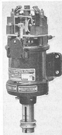
Abb. 5. Hauptstromzeitrelais.
