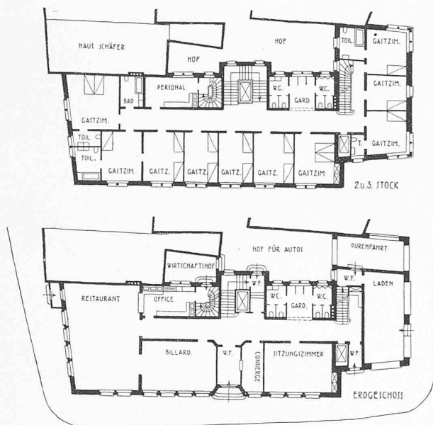
Grundrisse des neuen Hotels. — Masstab 1 : 500.
