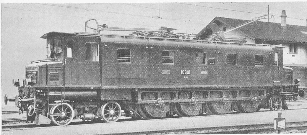
Abb. 1. A^{e4/7} Lokomotive mit BBC-Einzelachsantrieb der Schweizerischen Bundesbahnen.
