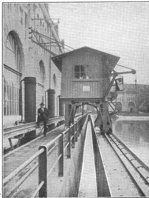
NORDOSTSCHWEIZ. KRAFTWERKE A.-G. BADEN. KRAFTWERK BEZNAU Kombinierte Rechen-Reinigungsmaschine mit doppeltem Schwenkkran und Geschwemmels-Abfuhrkanal
