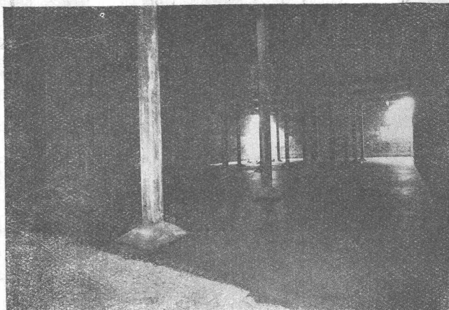
Reservoir, das infolge grosser Setzungsrisse und Porosität undicht war und nach unserm System mittels Dilatationseinlagen und durch Sika-4-Zement-Anstrich stabilisiert und gedichtet wurde.
