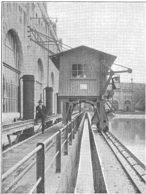
NORDOSTSCHWEIZ. KRAFTWERKE A.-G. BADEN. KRAFTWERK BEZNAU Kombinierte Rechen-Reinigungsmaschine mit doppeltem Schwenkkran und Geschwemmselfuhrkanal
