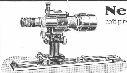
Kippregel Wild — 1/4 nat. Grösse
