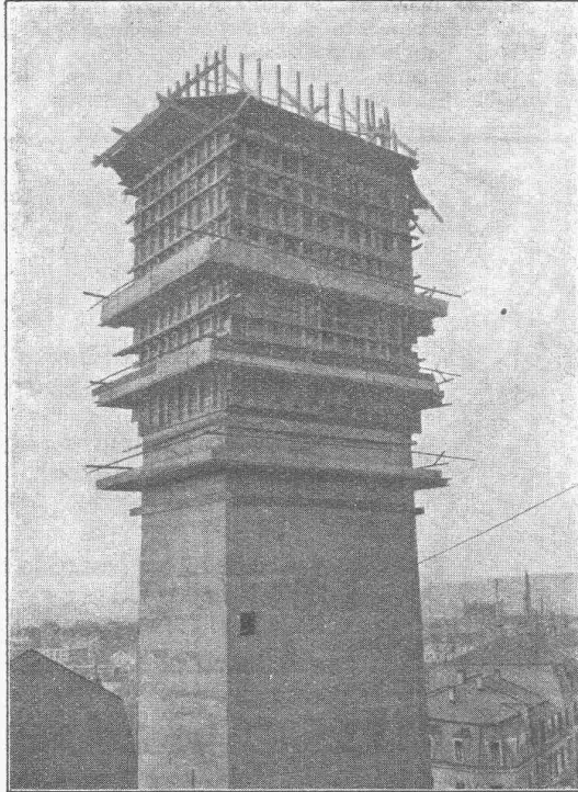
St. Antoniuskirche, Basel. Kirchturm in Eisenbeton.
