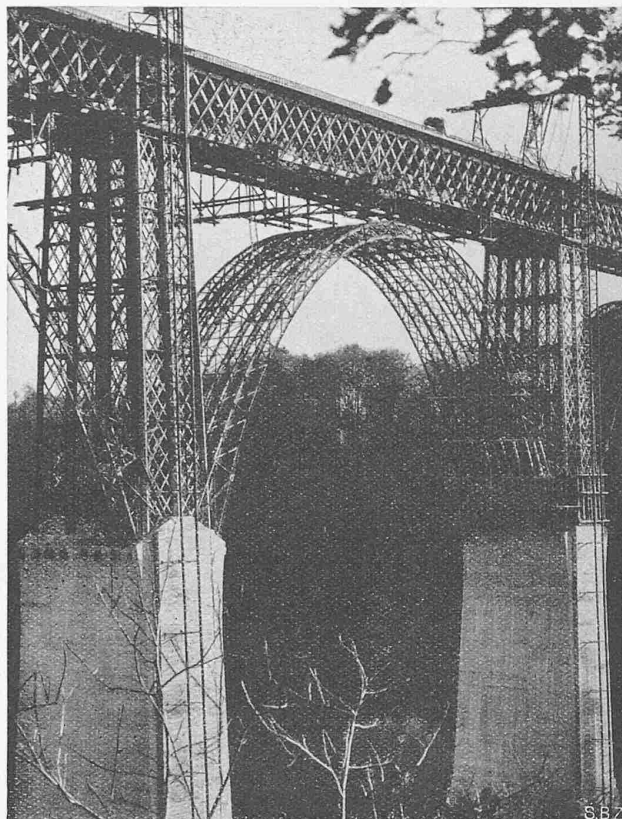
Abb. 4. Fertig montierte Melanbogen, links Montagebeginn (Aufn. 26. Okt. 1925). Hängegerüste mit dem Gitterträger, längs der Pfeilergerüste die Betonauflage. Melan-Konstruktion von Löhle & Kern A.-G., Zürich.
