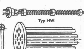
Einzelne elektrische Heizinsätze zum Einbauen.
