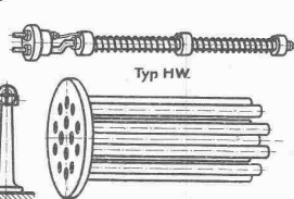
Einzelne elektrische Heizansätze zum Einbauen.
