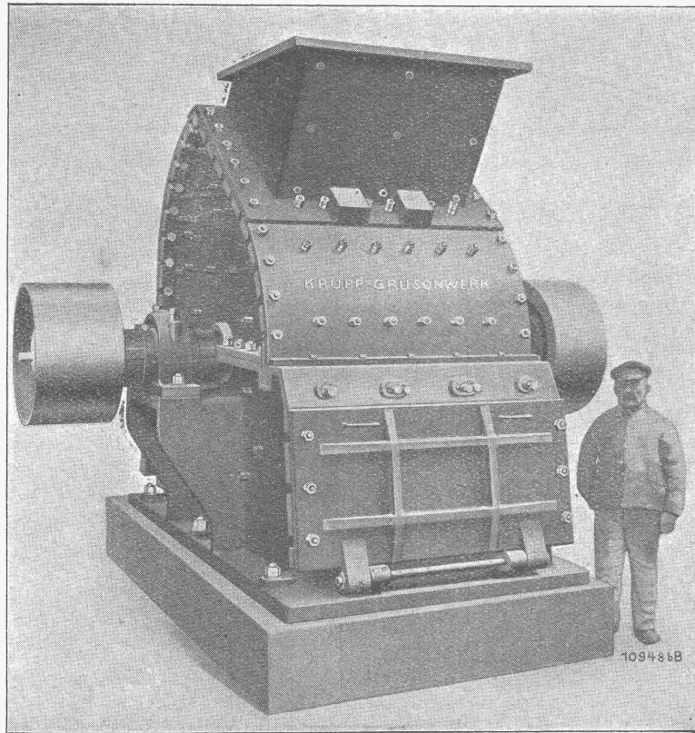
Hammerbrecher
