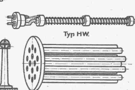
Einzelne elektrische Heizeinsätze zum Einbauen.
