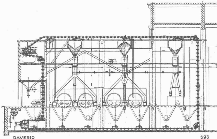
Ausgeführte Conveyor-Anlage in einem grossen schweiz. Industrie-Etablissement.
