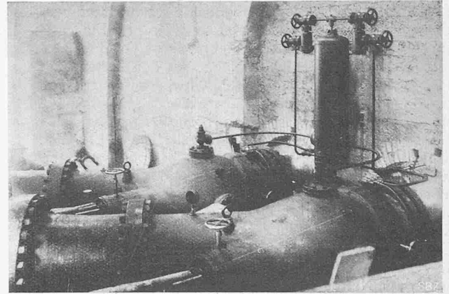
Abb. 85. Glockenschieber, Bauart Piccard, Pictet & Cie., der Turbinen 1 bis 5 des ersten Ausbaues.
