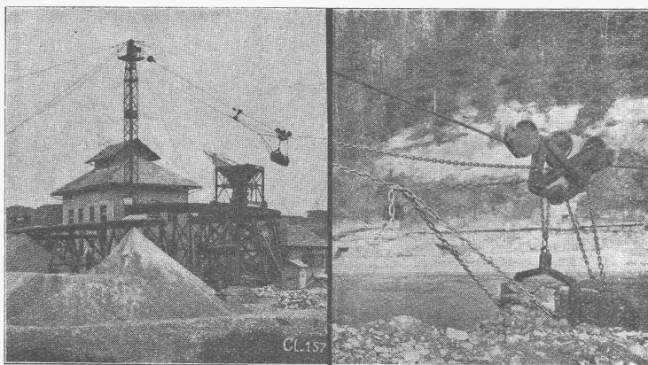
Kabelbaggeranlage, geliefert an die A.-G. für Sand- und Kiesverwertung Laupen.
