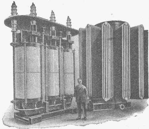
Drehstrom-Oeltransformator von 13000 kVA, mit Oelkühlung 70000/13500 Volt
