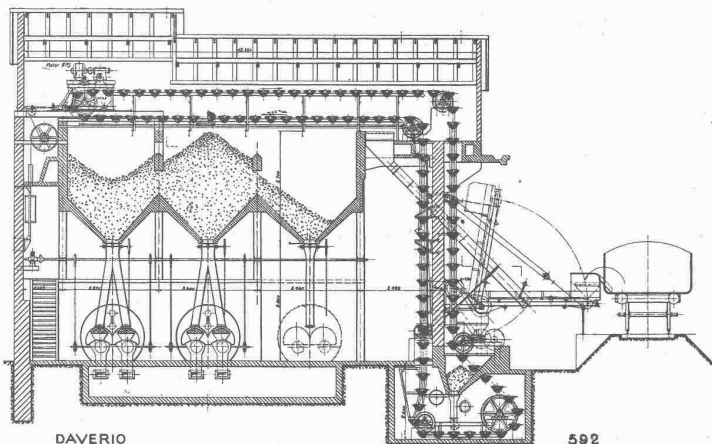
DAVERIO Ausgeführte Conveyor-Anlage in einem grossen schweiz. Industrie-Etablissement.
