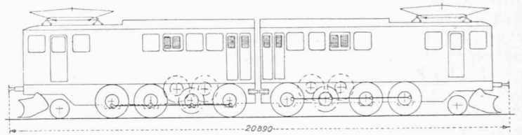
Abb. 6. Schwedische Staatsbahn (Kiruna-Riksgränsen). — Typ 1-C+C1.
