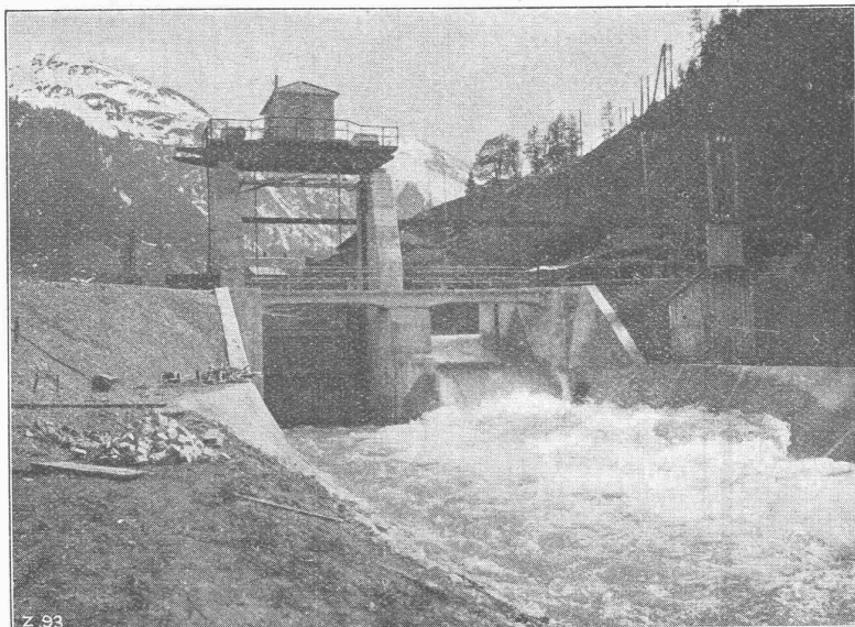
Wasserfassung des Kraftwerks Klosters-Küblis Ausgeführt 1920/21.
