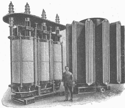
Drehstrom-Oeltransformator von 13000 kVA, mit Wasserkühlung 70000/13500 Volt
