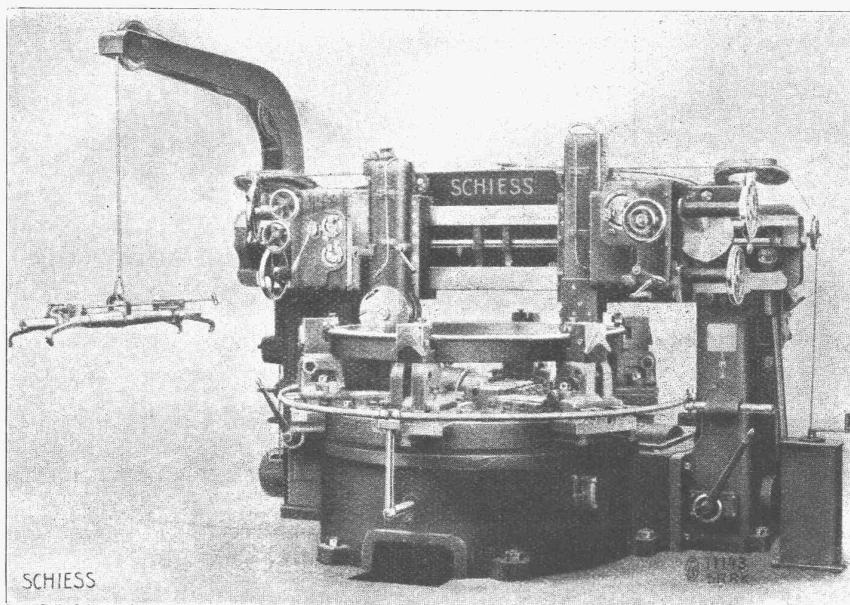
Radreifen-Bohrbank zum Ausbohren von Radreifen mit kleinen, mittleren und grossen Durchmessern. Planscheibe mit ausziehbaren Spannbalken.
