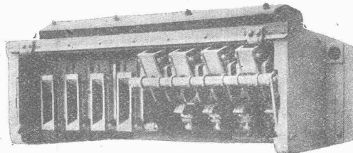
Batterie von acht elektro-pneumatischen Einzelschaltern für die Steuerung von zwei Motoren von 200 PS Gesamtleistung bei 750 Volt (Verschaltung weggelassen).
