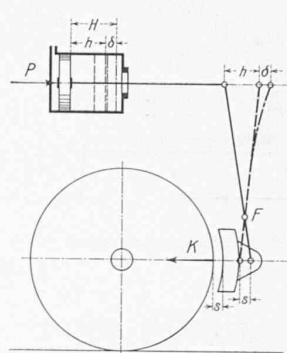
Abb. 13. Schema eines Bremsgestänges mit festem Übersetzungsverhältnis.
