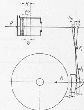
Abb. 14. Schema eines Bremsgestänges mit veränder- lichem Übersetzungsverhältnis.
