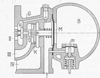
Abb. 12. Schematischer Schnitt des Božic-Steuerventils.
