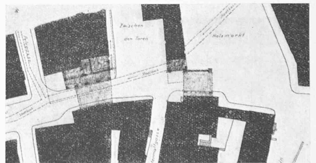
Entwurf Nr. 9 „Alt und neu“. — Situationsplan 1:1000.
