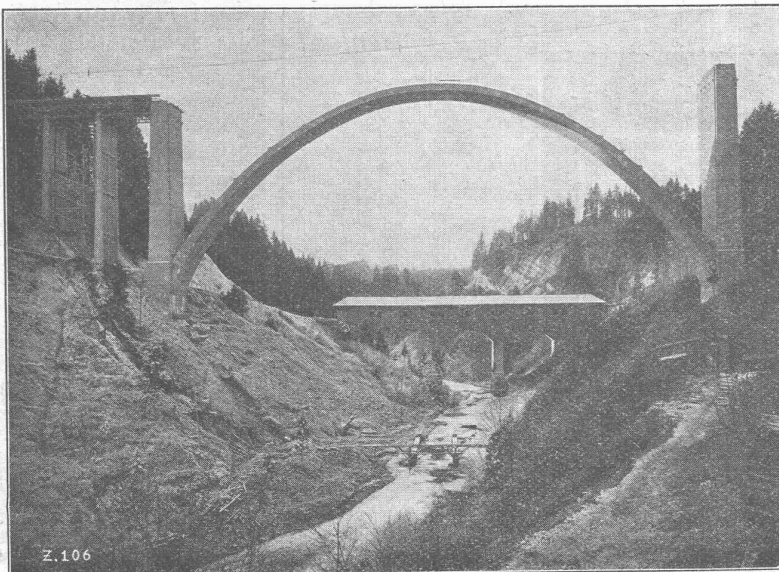
Hundwilertobelbrücke bei Waldstatt (Kt. Appenzell A.-Rh.) Eisenbetonbogen von 105 m Spannweite,
