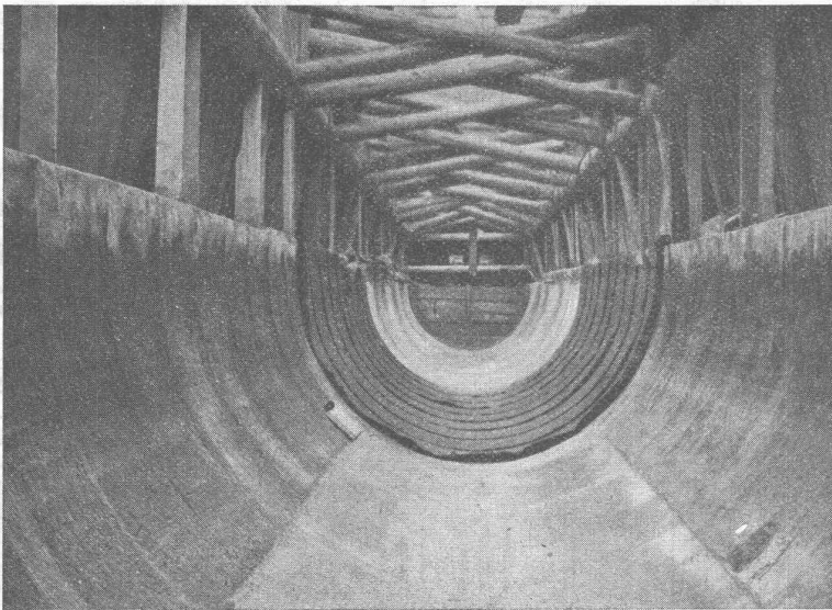
Bündnerische Kraftwerke A.-G.: Heberleitung in Klosters (330 m lang) Bauleitung: R. Moor, Ingenieurbureau, Zürich | Wasser- und luftdichte Isolation des Heberrohres mit „Mammut“ . . . . . 3000 m 2 Unternehmung: Locher & Co., Zürich Ausgeführt durch Asphalt-Emulsion A.-G.
