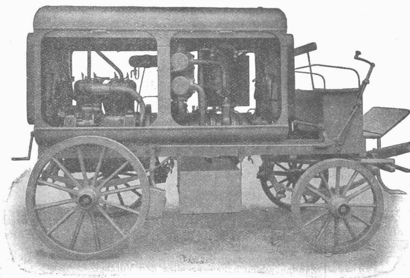
Fahrbare Kompressor-Anlage
