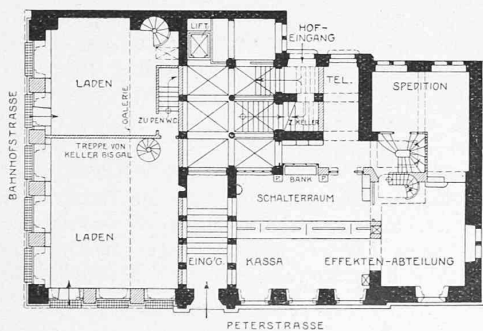
Entwurf „Lasius“. Schnitt und Grundrisse vom Erdgeschoss und 1. Stock. Massstab 1 : 400.
