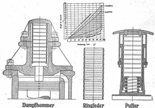
Dampfhammer
