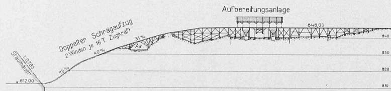
Abb. 10. Schnitt durch Aufbereitungsanlage, Silos, Betonmischer und Betoniereinrichtung. — Masstab 1 : 2000.
