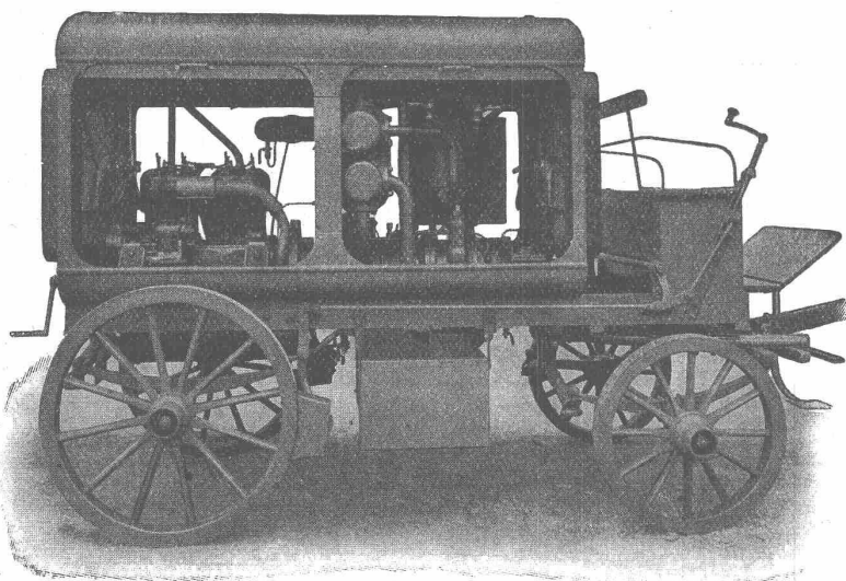
Fahrbare Kompressor-Anlage
