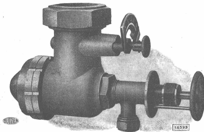
Oelbrenner: Leistung = 40 kg/Std.
