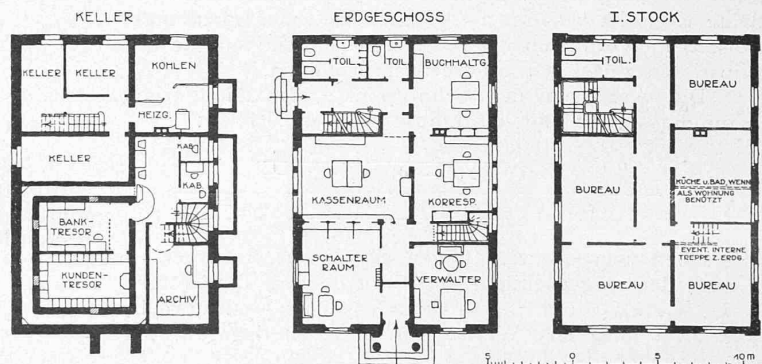
III. Preis (600 Fr.), Entwurf Nr. 1. Verfasser: Wilh. Brodbeck, Arch., Liestal. Grundrisse 1:400, Schaubild rechts nebenan.
