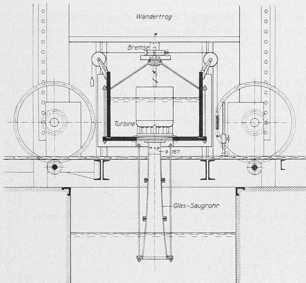
Abb. 17. Versuchseinrichtung in Kriens für die kleine Modellturbine ( D_s = 167 mm) mit geradem Glas-Saugrohr. — 1 : 50.
