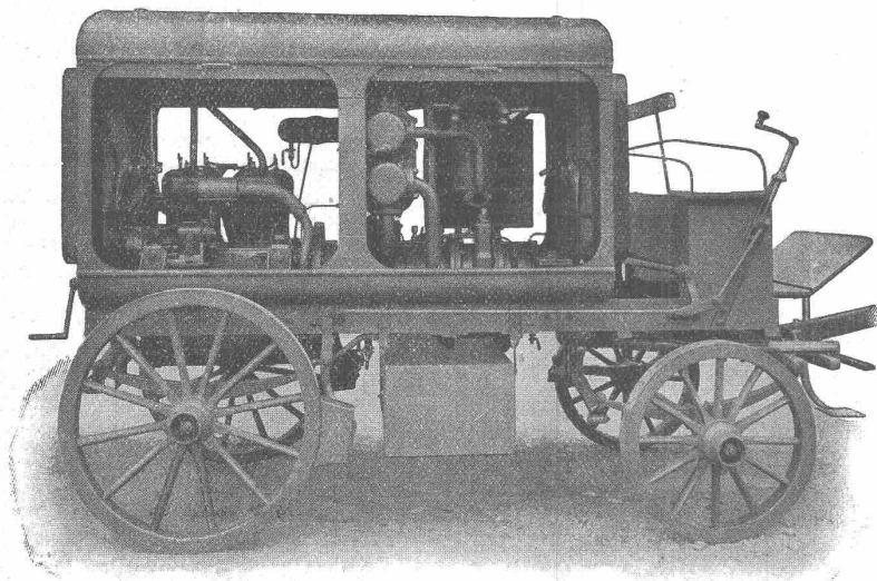
Fahrbare Kompressor-Anlage
