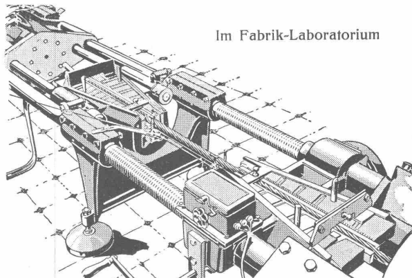
Drahtseil-Zerreiss-Versuch
