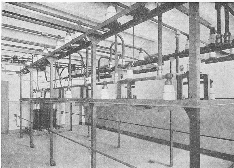
Abb. 18. Sammelschienen für 15 kV im Zwischenstock.
