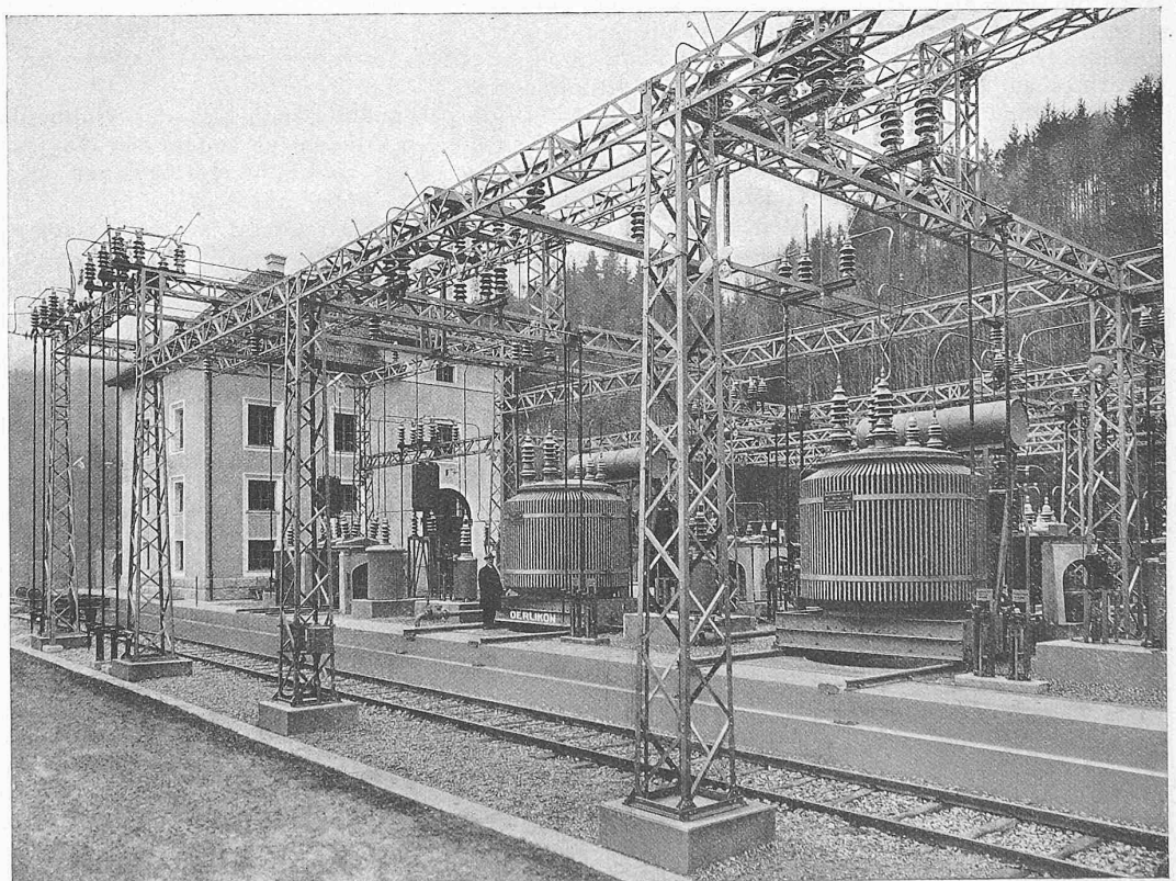
Abb. 5. Blick auf die Transformatoren, dahinter die 15 kV Schalter; links ein 60 kV Schalter.
