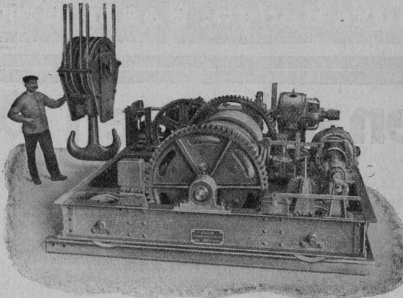
Chariot d'un pont roulant de 50 tonnes.
