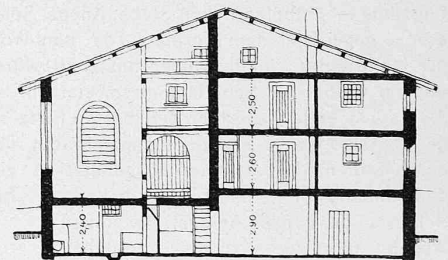
LANGSSCHNITT
