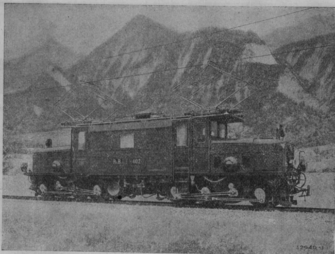
Einphasenstrom-Lokomotive, Type C-C für die Rhätische Bahn 2×600 PS, 10 000 Volt, Fahrdrahtspannung 16\frac{2}{3} Per/sec Geschwindigkeit 30 bis 45 km/h, Spurweite 1 m.
