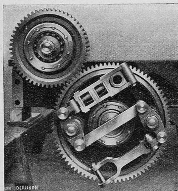
Abb. 7. Einzelachsantrieb „Oerlikon“.
