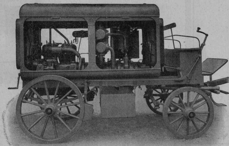
Fahrbare Kompressor-Anlage
