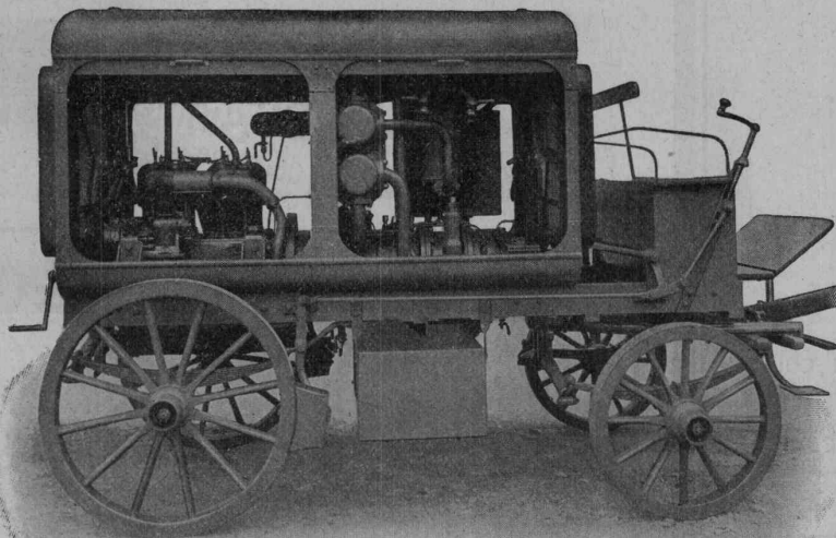
Fahrbare Kompressor-Anlage
