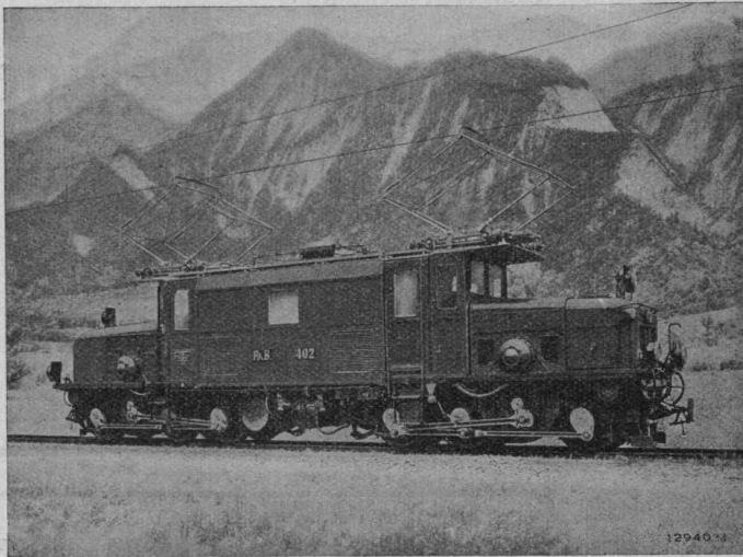
Einphasen-Schnellzuglokomotive mit Einzel-Achsantrieb Type 2-C-1 für die Schweizerischen Bundesbahnen, 3 \times 700 PS, 15000 Volt Fahrdrachtspannung, 16\frac{1}{3} Per/sec, max Geschwindigkeit 60 bis 90 km/h.
